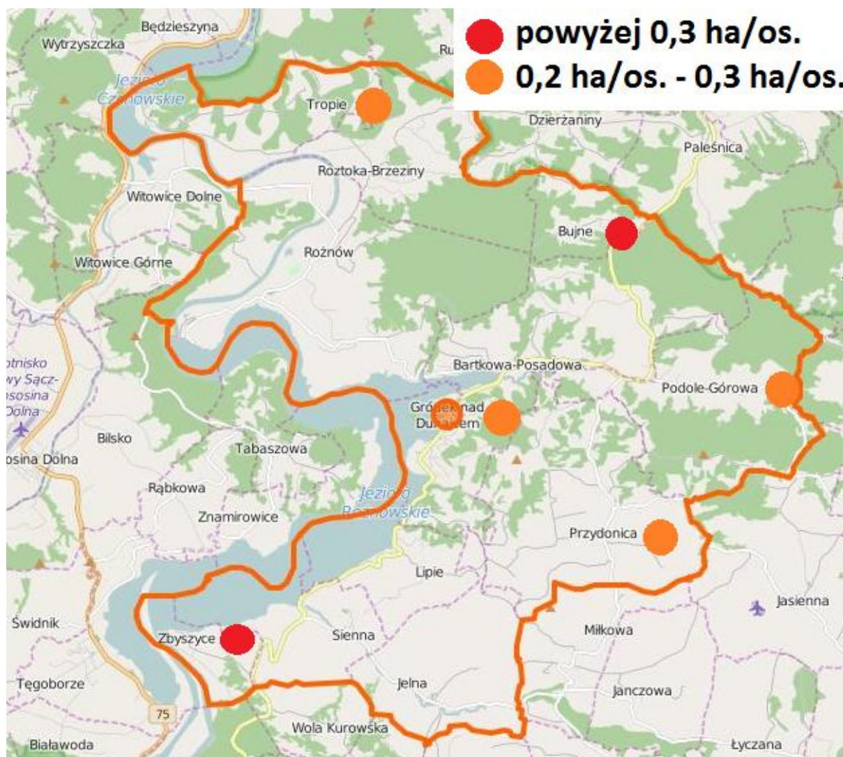
Rysunek 15. Miejsca na terenie Gminy Gródek nad Dunajcem o najwyższych wskaźnikach występowania zjawiska osuwisk ziemi
